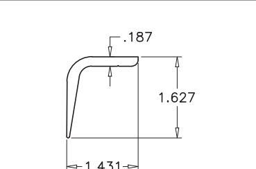
9 ASTRAGAL
