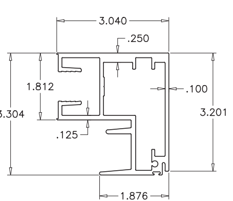
8 INTERLOCK STILE
