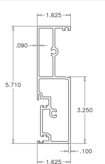
3 FRAME JAMB
