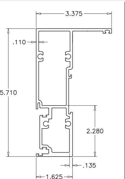
33 OXO LOCK STILE
